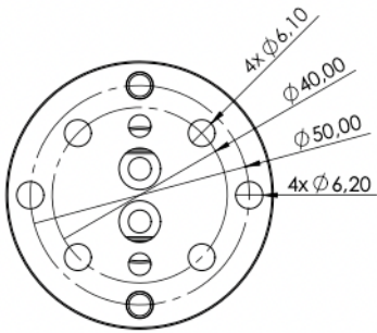
Robot Adapter ISO 9409-A50 Art.No. SG.AN.R50
